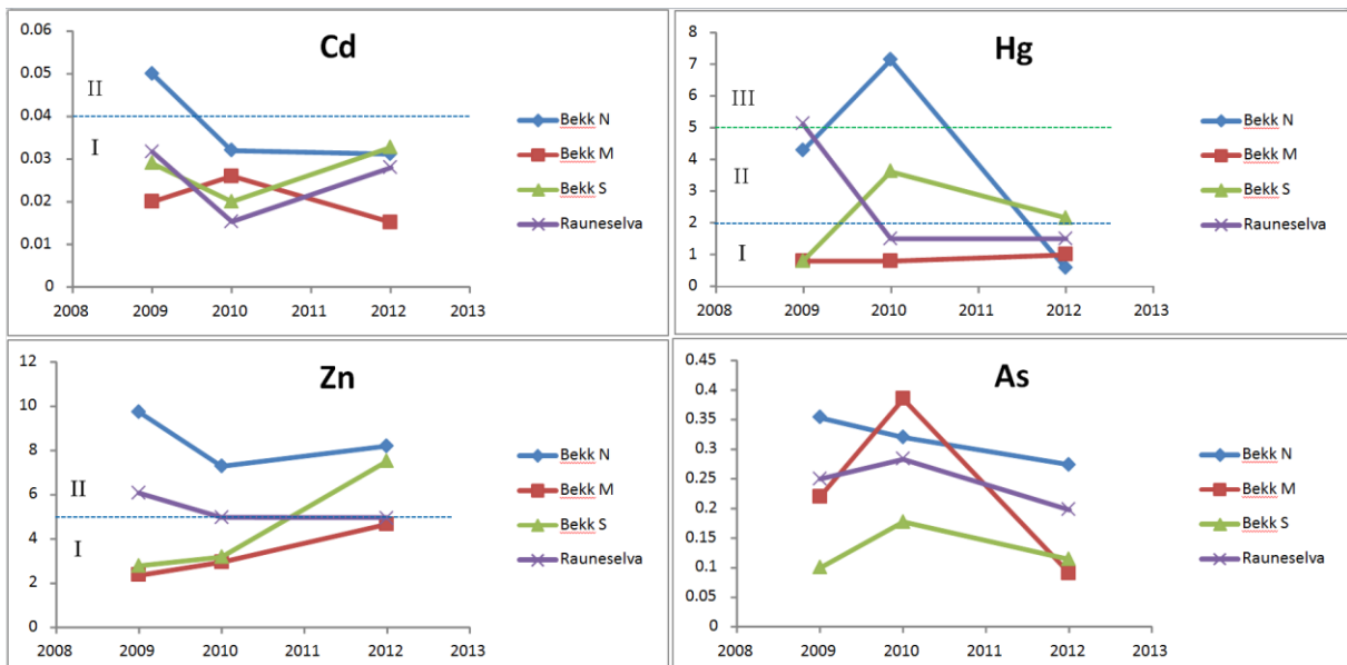
Figur 7: Middelmiddelkonsentrasjon av kadmium (Cd), kvikksølv (Hg), sink (Zn) og arsen (As) i fire vannveier gjennom anleggsområdet på Raunes i perioden 2009-2012. Resultater fra nederste målepunkter vist. Konsentrasjoner er gitt i mikrogram/liter for Cd, Zn og As, og i nanogram/liter for Hg. X-aksen viser årstall. Grenseverdier for tilstandsklasse I (ubetydelig), II (moderat) og III (markert) forurensset etter klassifiseringsnøkkel TA-1468 er markert med stiplede linjer og romertall.
